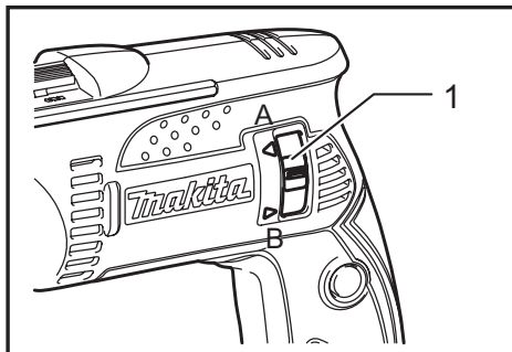
► 1. Interruptor de inversión
