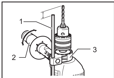
► 1. Calibrador de profundidad 2. Empuñadura lateral de mango 3. Base de la empuñadura
